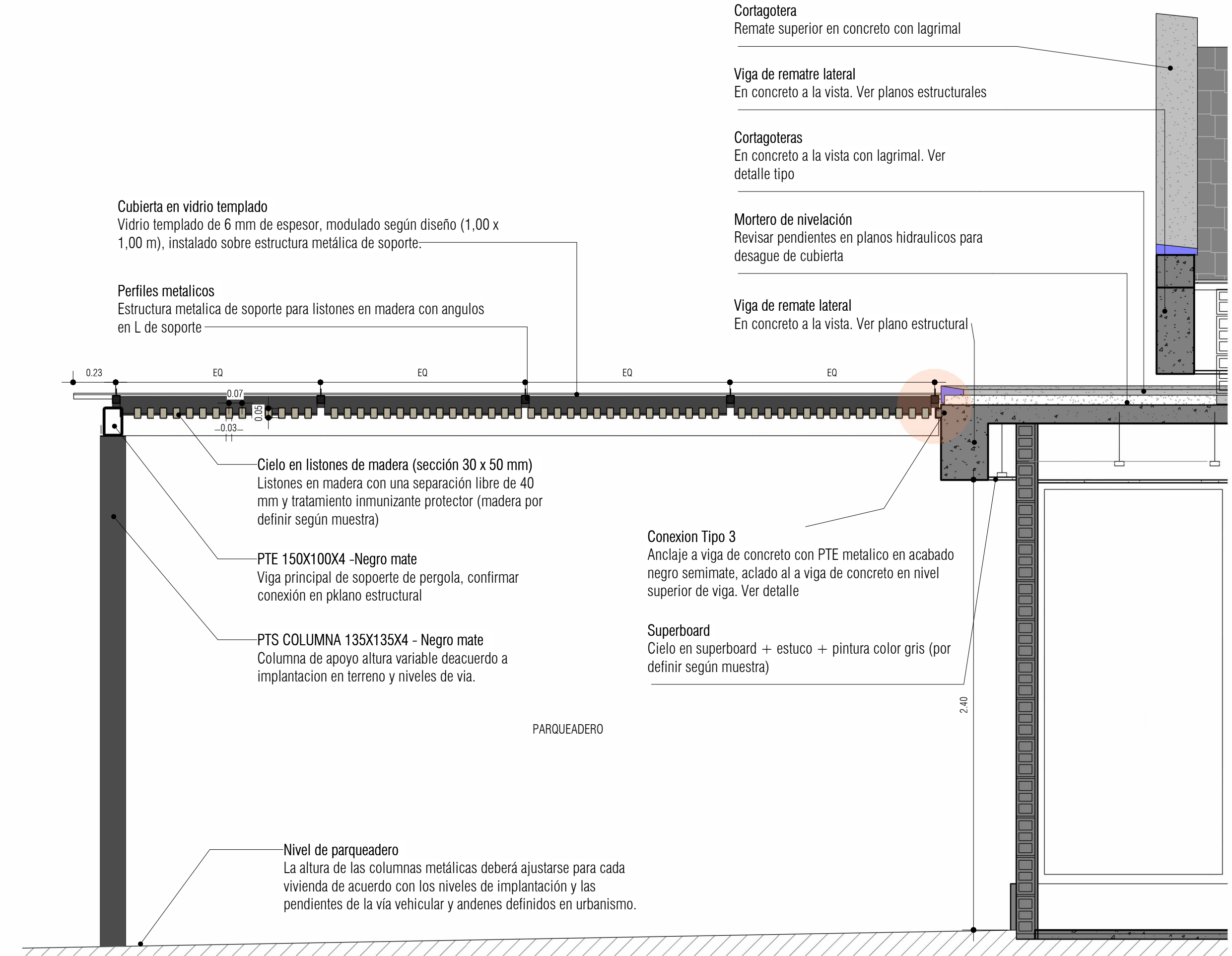
DETALLE PERGOLA PARQUEADERO 1:10
