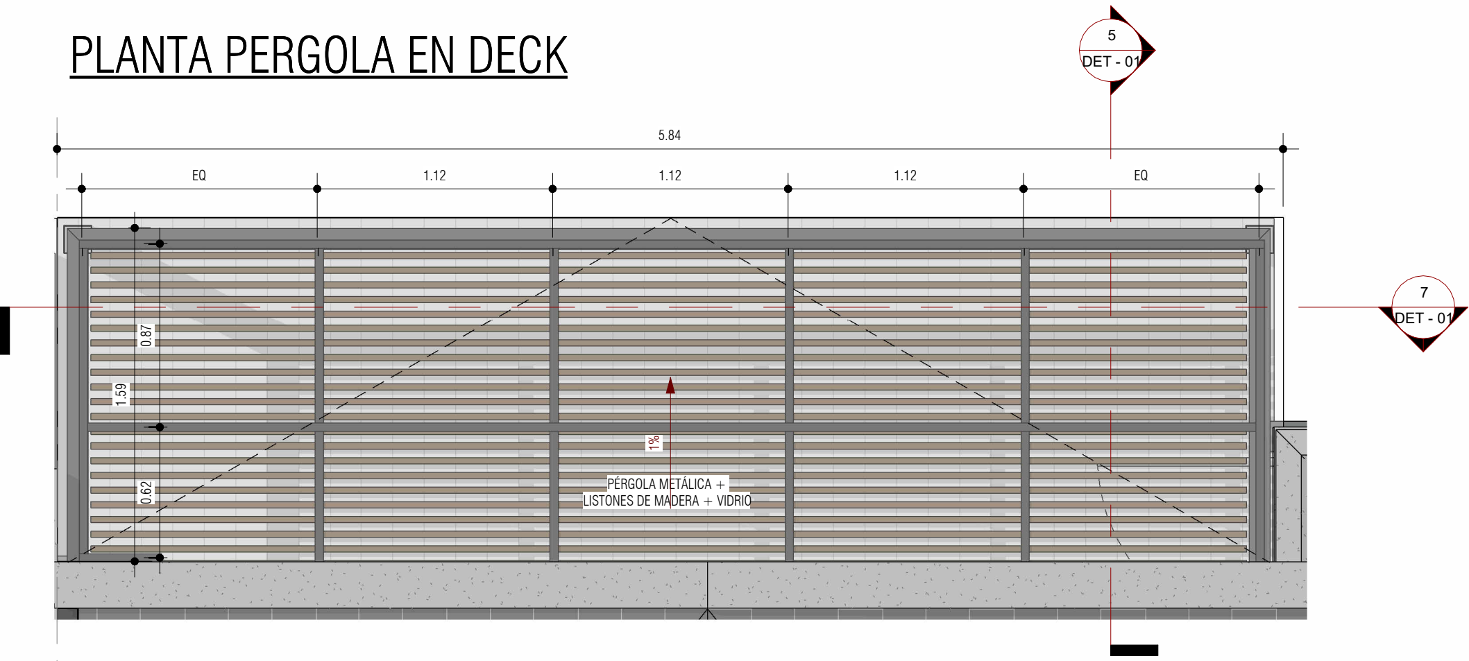
2 PERGOLA DECK - CASA 16 1:25
