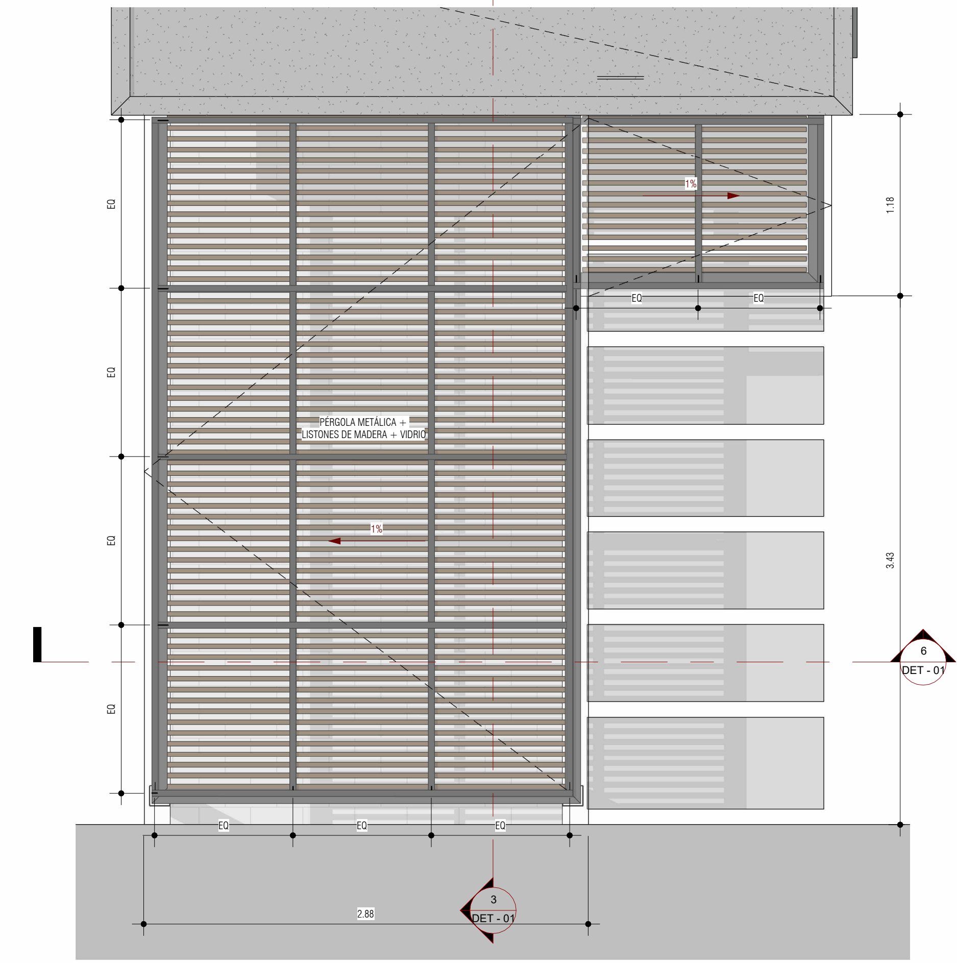
4 PERGOLA PARQUEADERO - CASA 16 1:25
