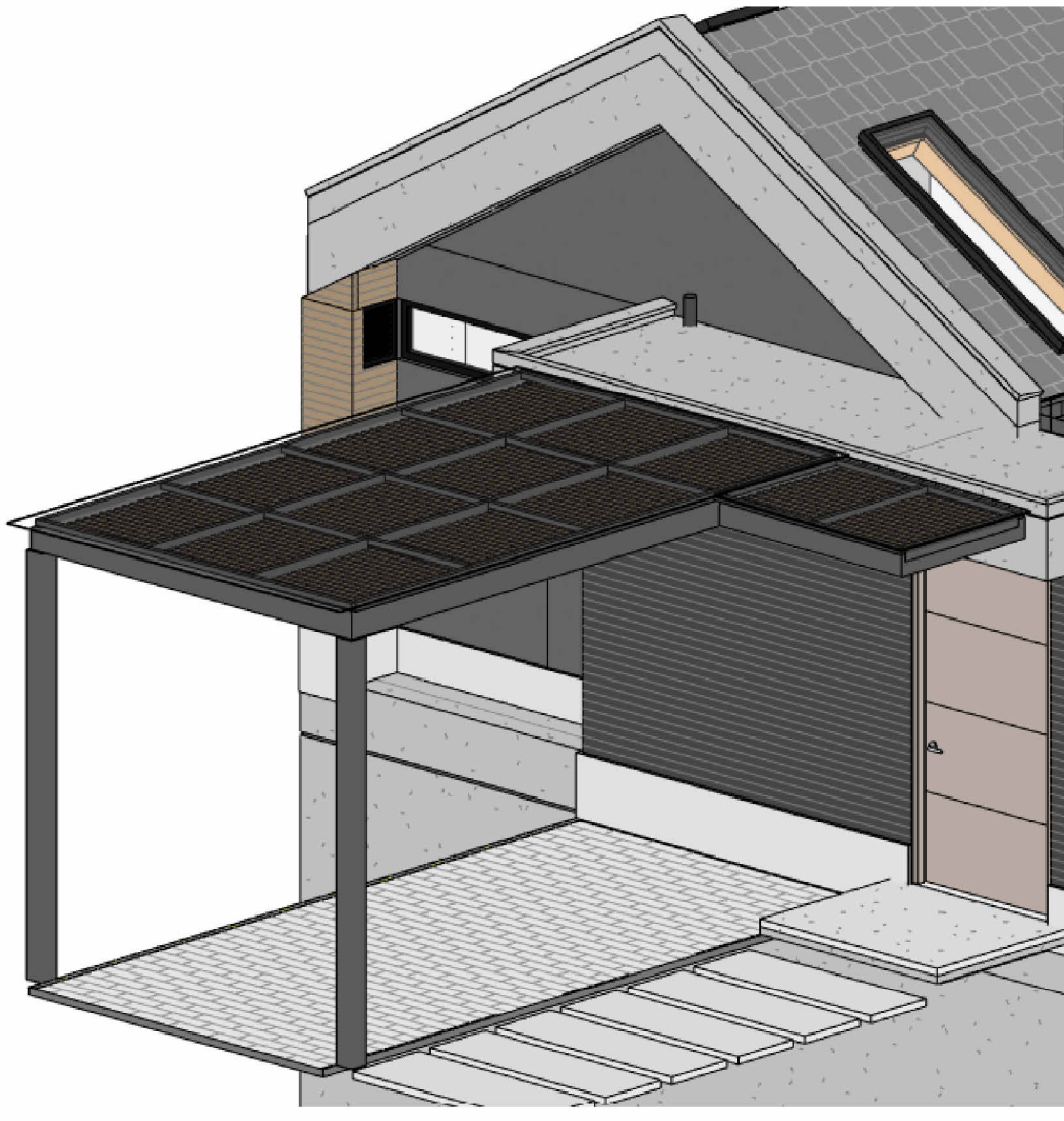
Imagen de referencia Pergola parqueadero + ingreso peatonal
