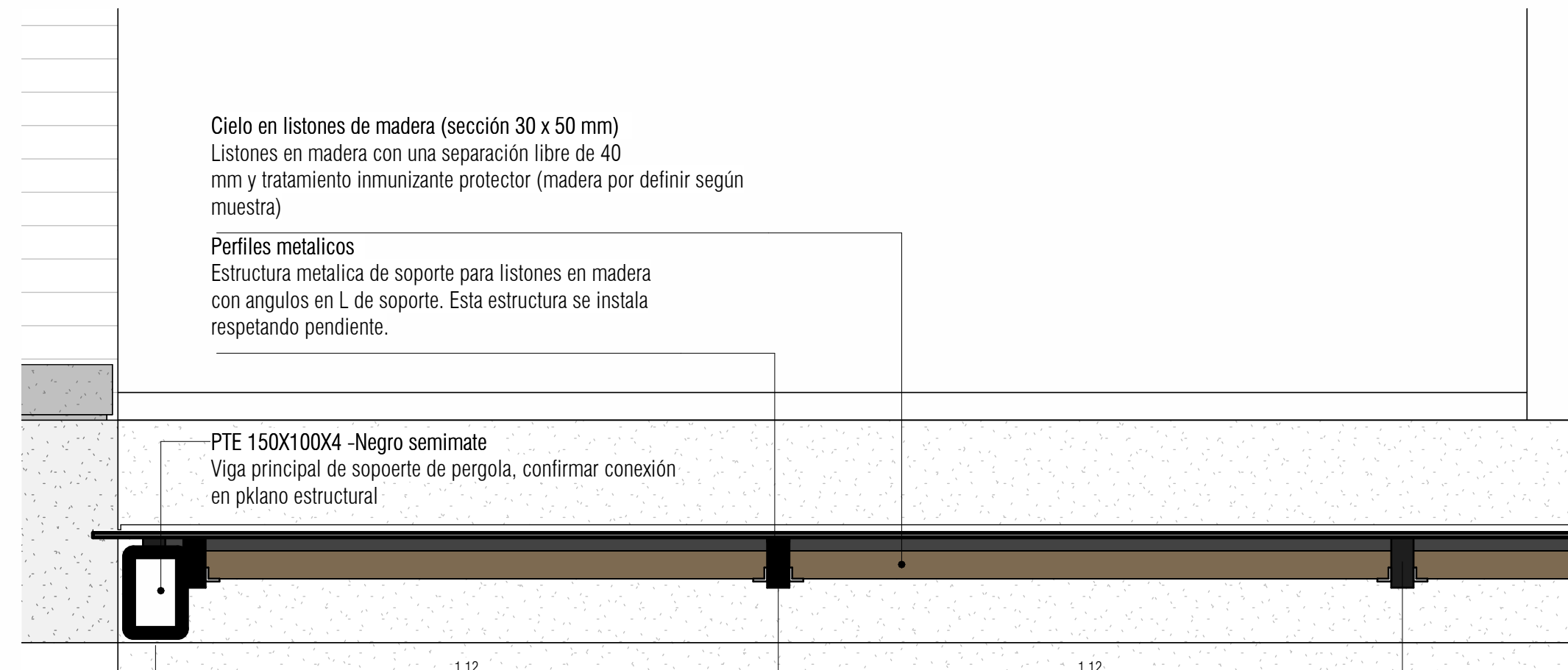
7 CORTE FACHADA PERGOLA DECK - DET-01 1:10
