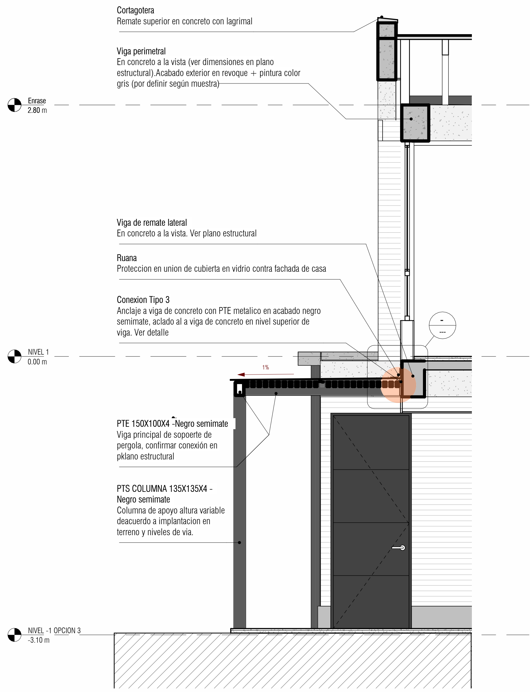
5 SECCIÓN TRANSVERSAL PERG. DECK 1:25
