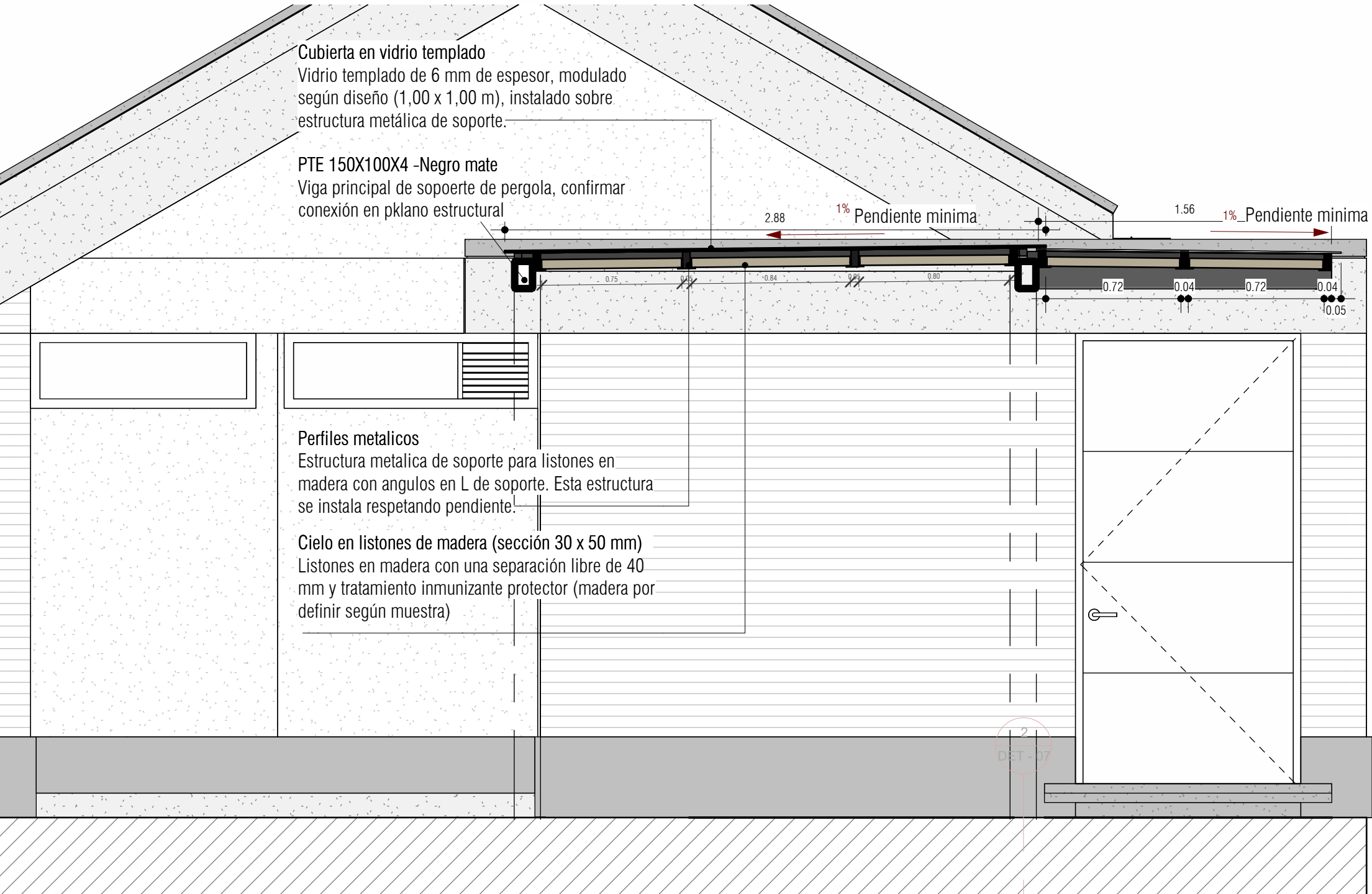
6 CORTE POR FACHDA TRANS - PERGOLA PARQUEADERO 1:25
